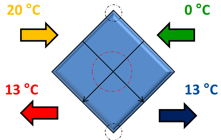
Перекрестный теплообменник КПД 65 %
